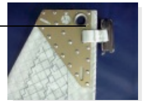
wysokowytrzymała nitowana głowica aluminiowa z ręcznie doszywanym pelzaczem
